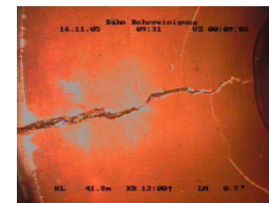
Schadensbilder aus der Kanalinspektion
